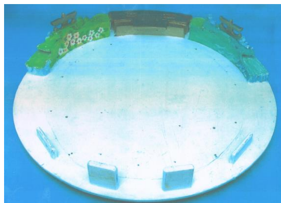
5-фигура. Полдун негизги көрүнүшү Фиг. 5. Вид основания пола
